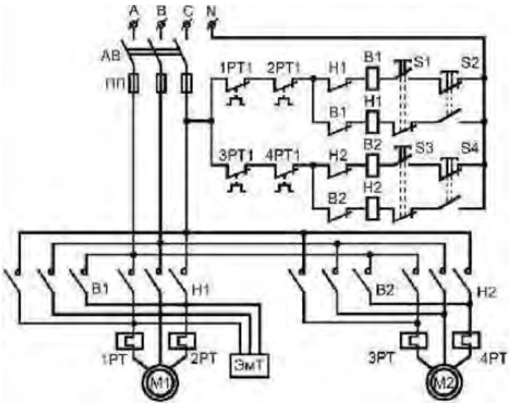
Электрическая схема управления электроталью AB-автоматический выключатель; B1,H1;B2;H2-контакты, S1,S2-кнопки «подъема» и «спуска»; S3,S4-кнопки «вперед», «назад»;ЭМТ-электромагнитный тормоз.
